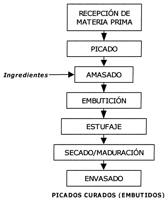
Figura 7. Diagrama de flujo y descripción de las operaciones del proceso de elaboración de productos picados curados.
